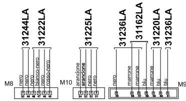
SCHEDA MODULAZIONE MICROCODE SM 20018 COD. 76662LA
